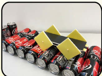
方輪車製作
